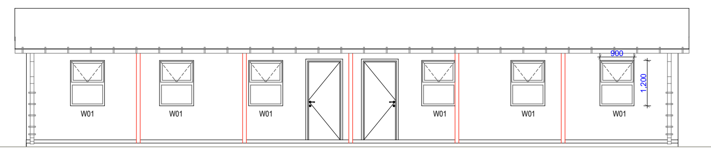
E-01 Elevation 1:100
